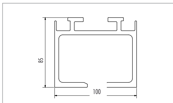
▲ DORRslide 1+2 ohne Auflagewinkel
