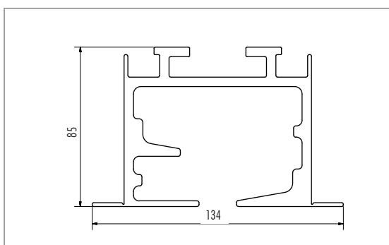
▲ DORRsilent mit Auflagewinkel
