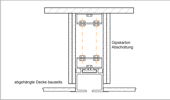
▲ Abhängung mit Abschottung
