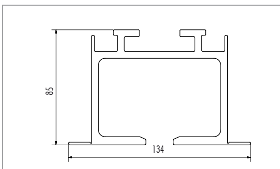
▲ DORRslide 1+2 mit Auflagewinkel
