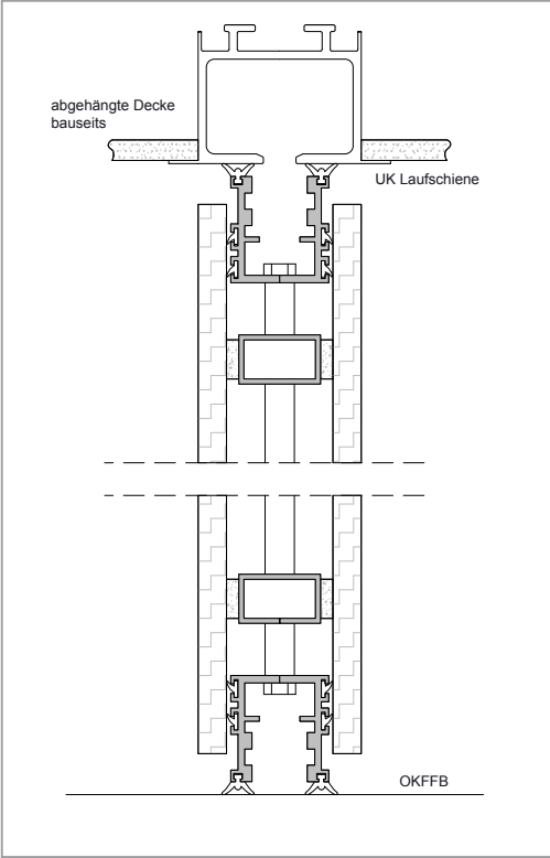
▲ Schnitt horizontal
