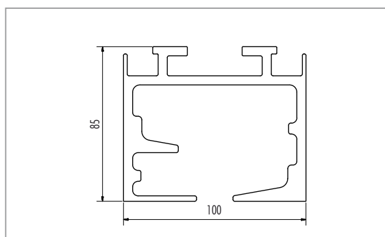
▲ DORRsilent ohne Auflagewinkel
