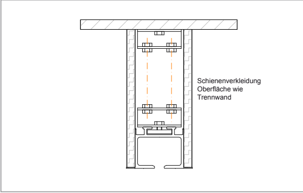
▲ Abhängung mit Laufschienenverkleidung
